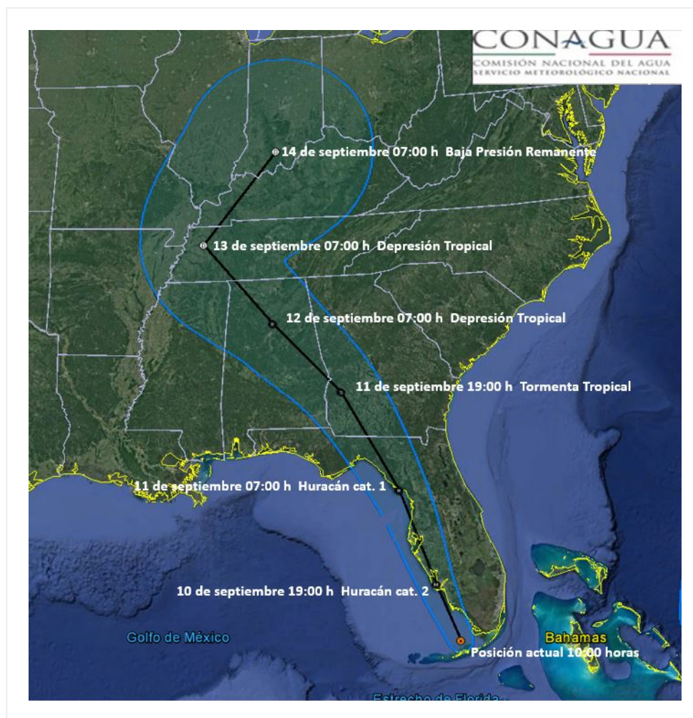
Trayectoria pronóstico del Huracán "Irma" cat. 4
